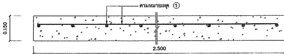
แบบขยายเหล็กตะแกรง 1:10
