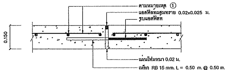
แบบขยาย EXPANSION JOINT 1:10
