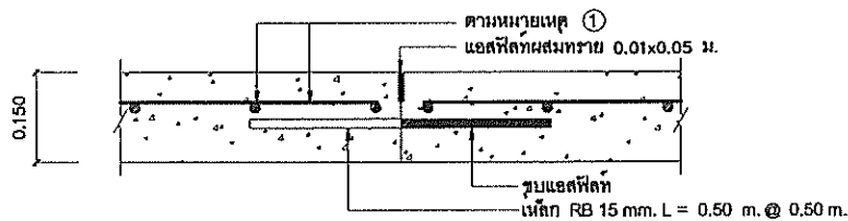
แบบขยาย CONTRACTION JOINT 1:10
